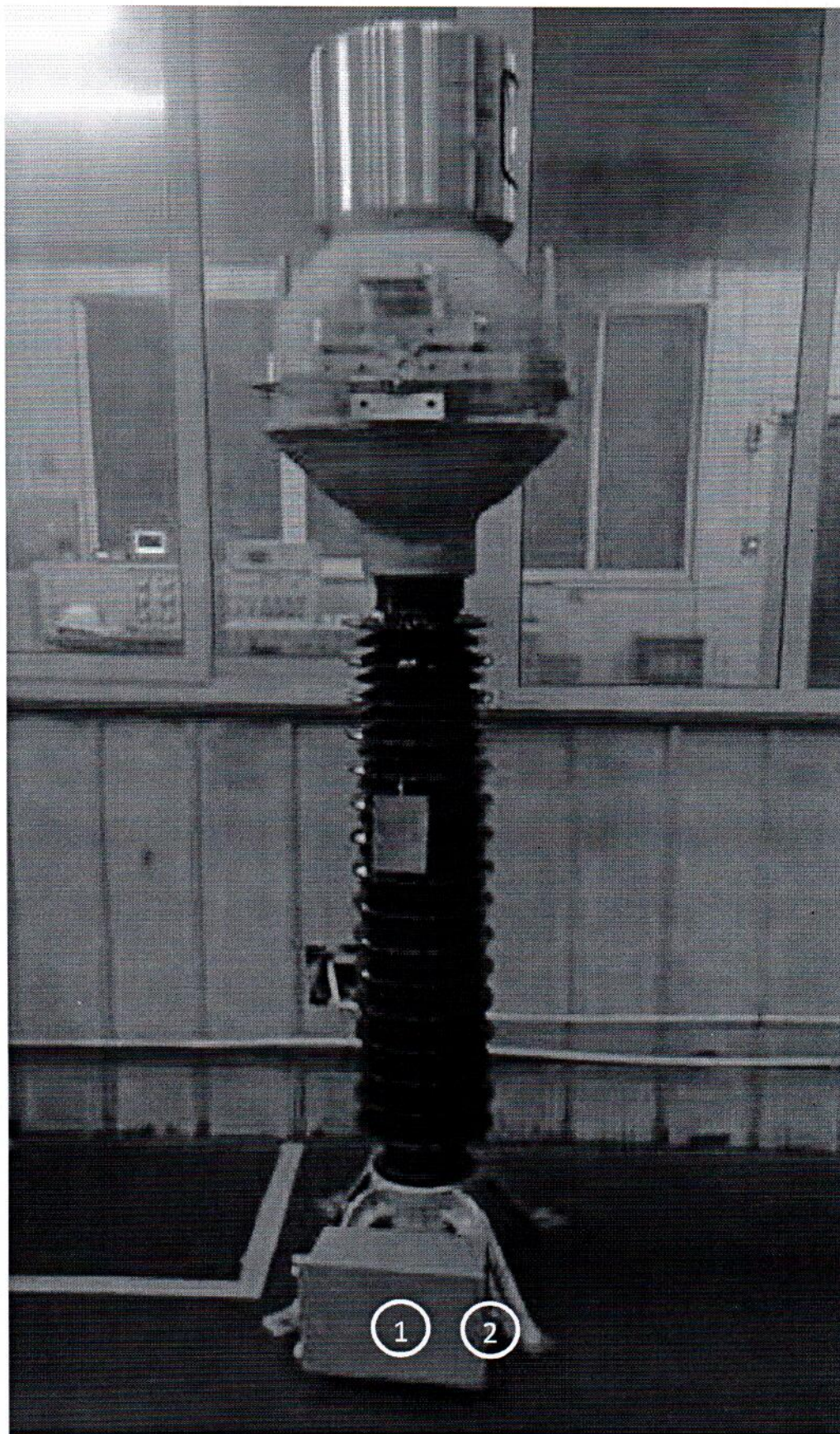
Рисунок 1 - Фотография общего вида со схемой нанесения знака поверки и места пломбировки 1 - место нанесения знака поверки, 2 - место пломбировки от несанкционированного доступа
