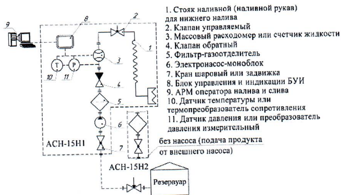
Рисунок 3 – Система измерительная нижнего налива: АСН-15Н1 (с насосом), АСН-15Н2 (без насоса). Измерительная схема
