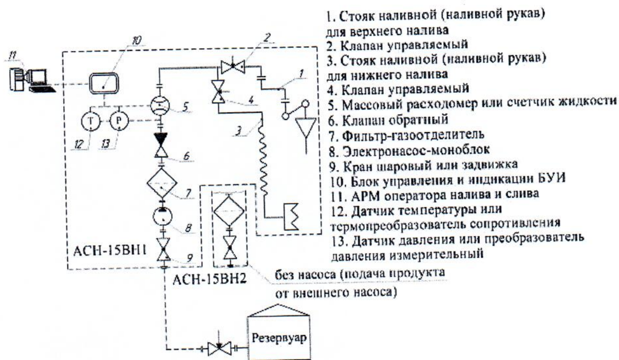
Рисунок 4 – Система измерительная комбинированного налива: АСН-15ВН1 (с насосом), АСН-15ВН2 (без насоса). Измерительная схема
