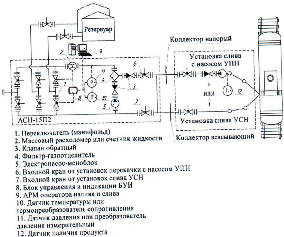
Рисунок 8 – Система измерительная для приёмки и перекачки продукта от ЖД цистерн в резервуары (групповой/поколлекторный учет) и между резервуарами АСН-15П2. Измерительная схема
