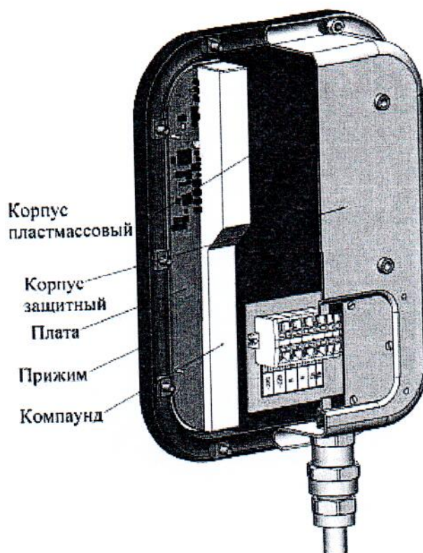
Рисунок 10 – Схема пломбировки БУИ от несанкционированного доступа
