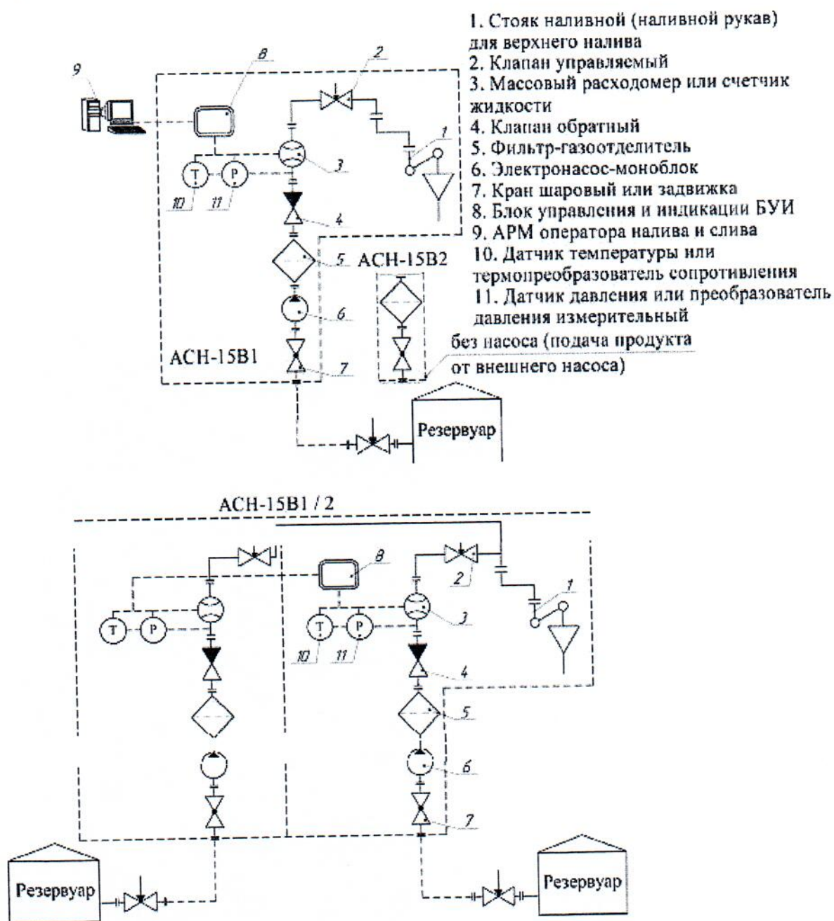
Рисунок 2 – Система измерительная верхнего налива: АСН-15В1 (с насосом), АСН-15В2 (без насоса), АСН-15В1/2 (с насосом). Измерительная схема
