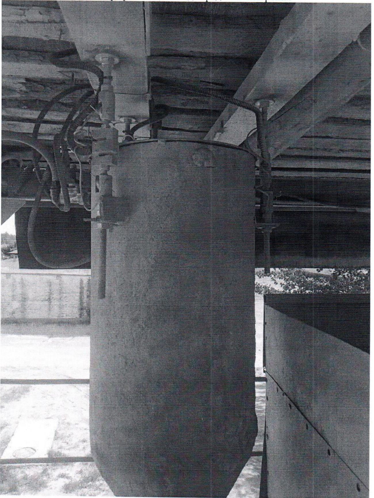
Рисунок А.1 – Внешний вид весов бункерных тензометрических ТВБв-150
