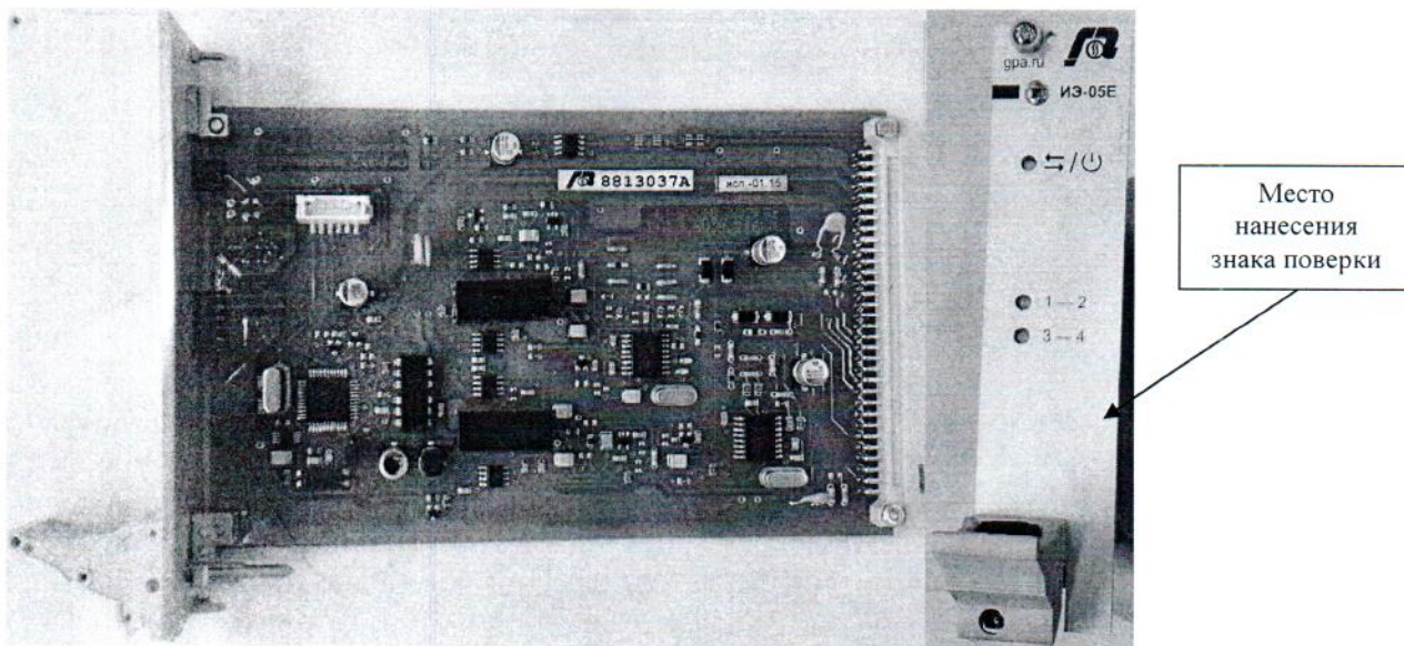
Рисунок 1 - Внешний вид печатной платы ИЭ-05Е
