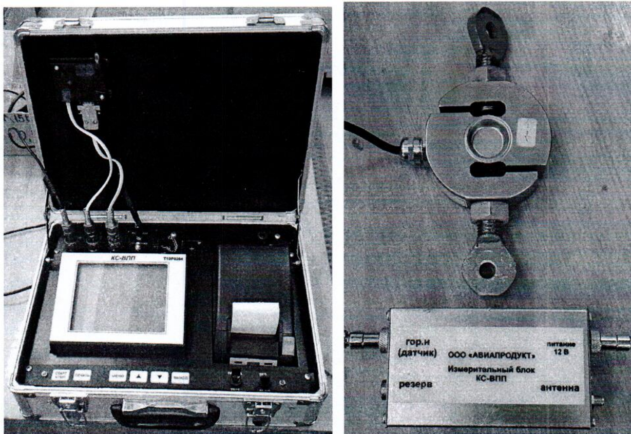
Рисунок 1 – Общий вид блока регистрации измерительного КС-ВПП
