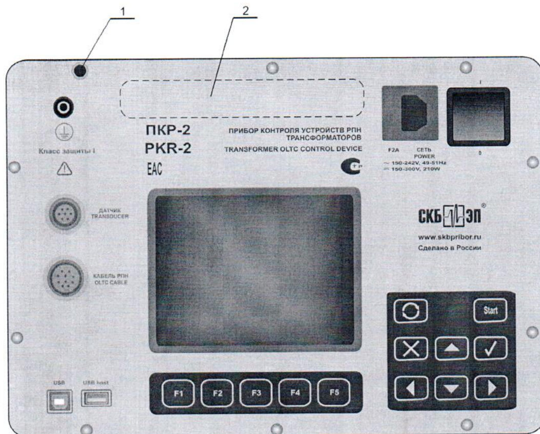
Рис. 3 Схема панели
