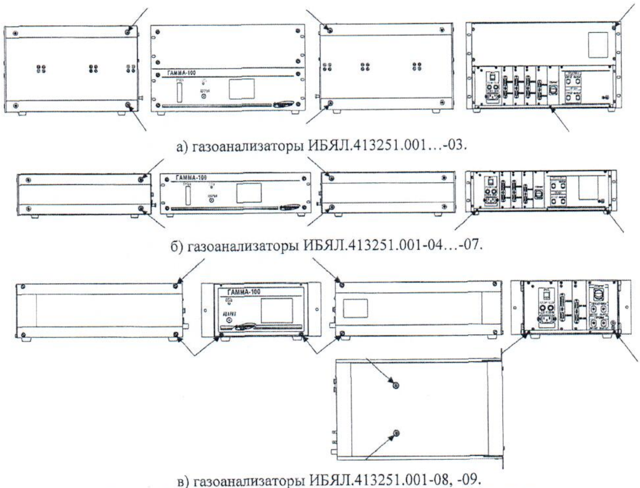
Рисунок 1 - Общий вид газоанализаторов ГАММА-100
