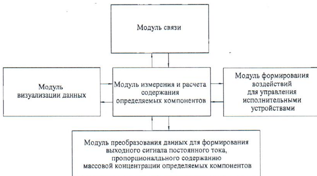
Рисунок 3 - Структура ПО
