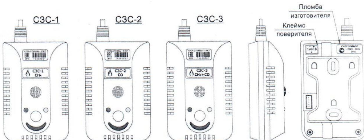
Рисунок 2 – Модификации и схема пломбирования
