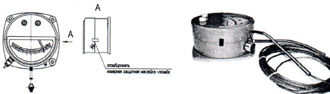
Схема пломбирования
