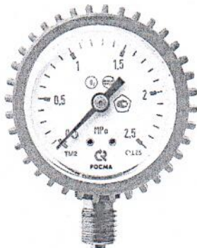
Рисунок 3 – Манометры показывающие ТМ, серия 10, газовые
