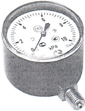
Рисунок 1 – Манометры показывающие KM, KV и KMB, серия 11
