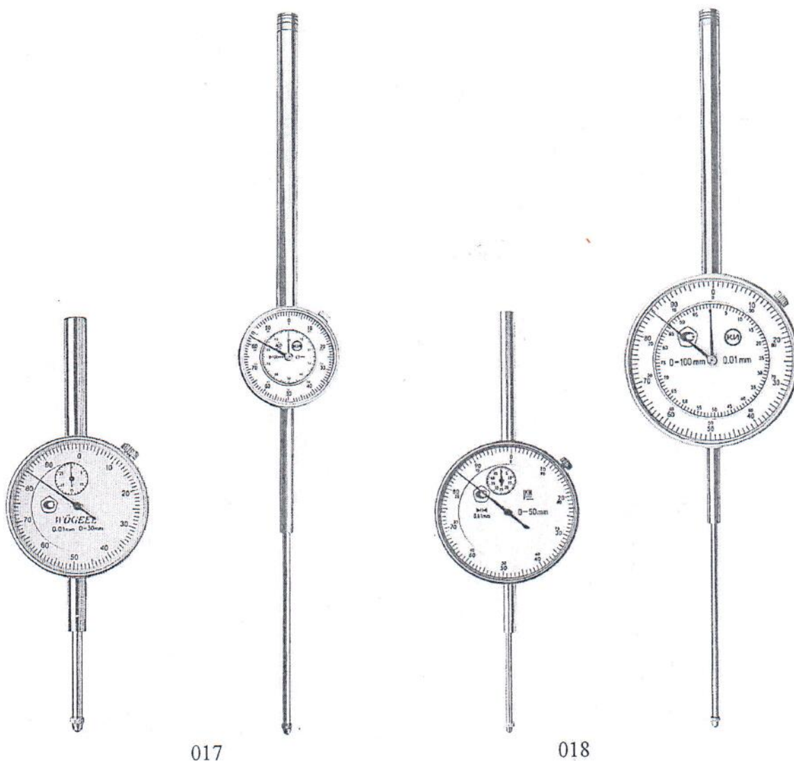
Рисунок 2 – Общий вид индикаторов ИЧ артикулы 017-018
