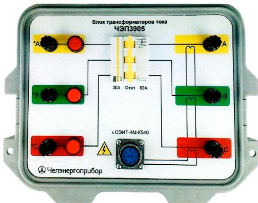
Рисунок 3- Внешний вид БТТ измерителя СЭИТ-4М-K540
