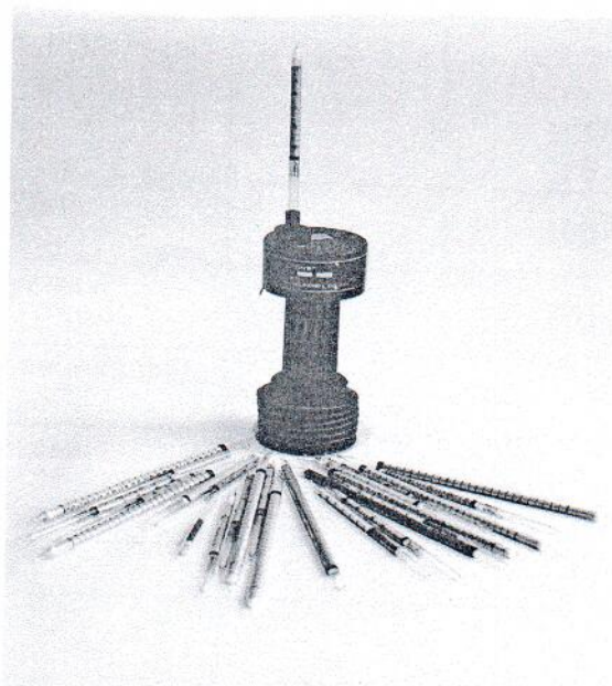
Рисунок 1 - Внешний вид трубок индикаторных С-3
