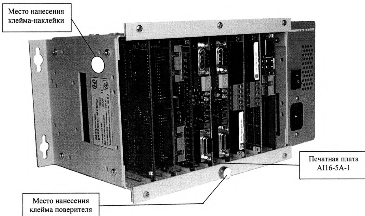
Рисунок 1. Внешний вид контроллеров
