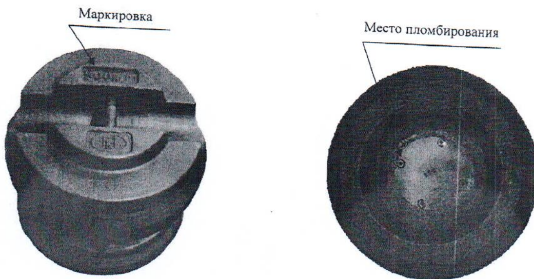
Рисунок 10 – Общий вид гири ГО-П-500 кг класса точности M_1 с указанием места пломбирования
