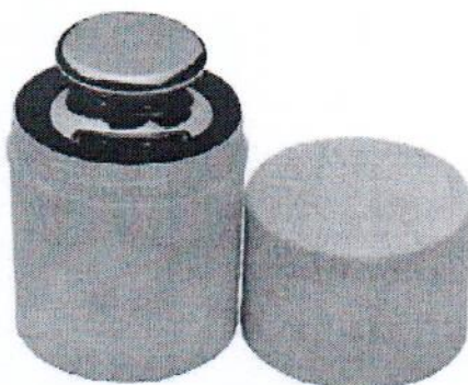
Рисунок 5 – Общий вид гири ГО-П-5 кг класса точности M_1
