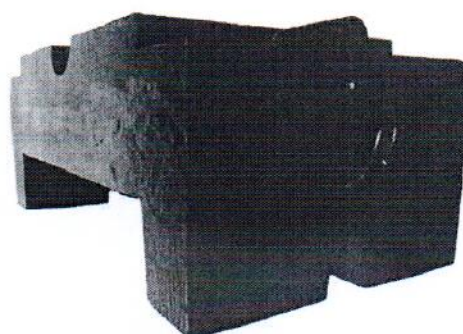
Рисунок 7 – Общий вид гири ГО-П-500 кг П класса точности M_1 с указанием места пломбирования
