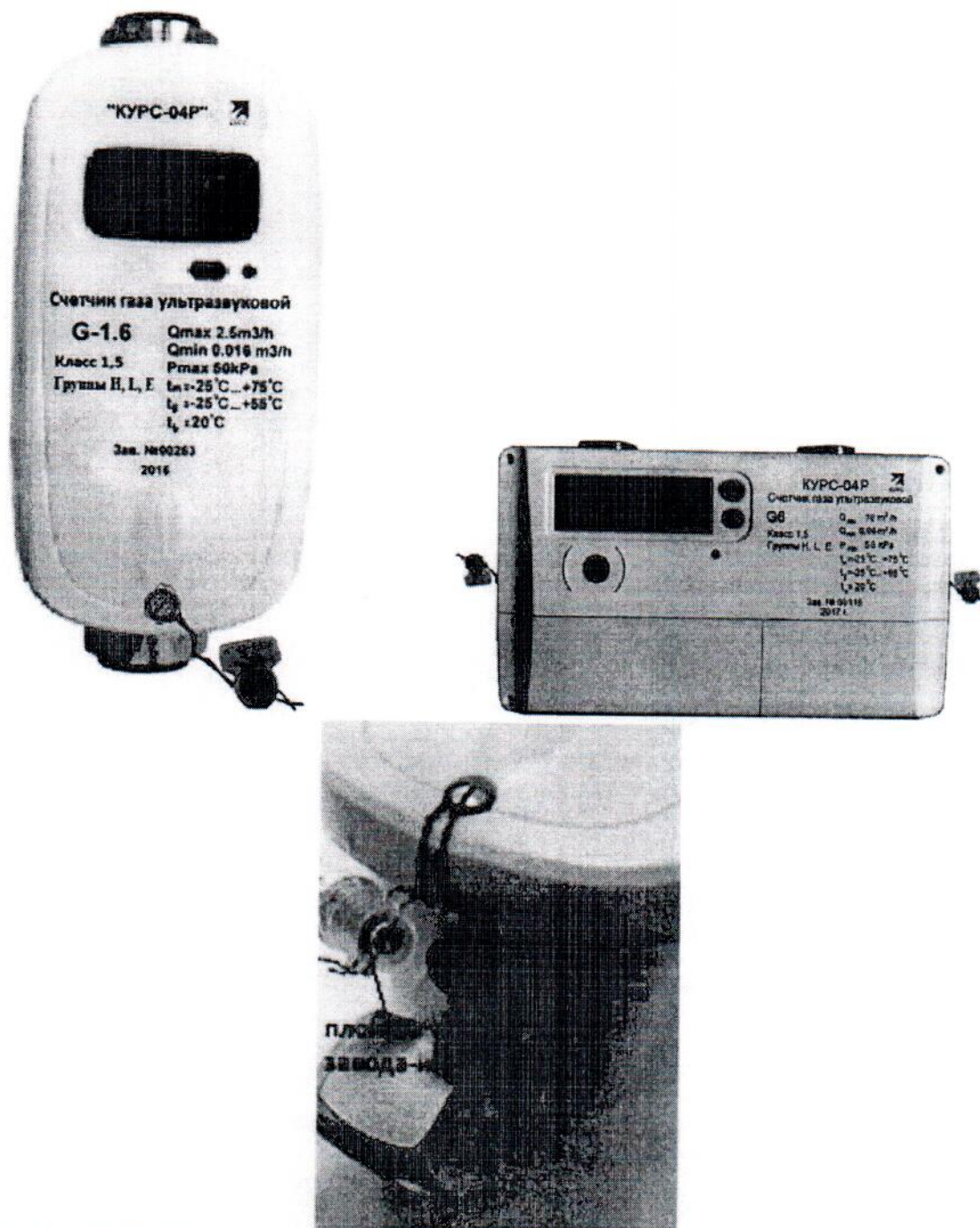
Рисунок 1 – Общий вид и схемы пломбировки от несанкционированного доступа счетчиков газа ультразвуковых «Курс-04Р»
