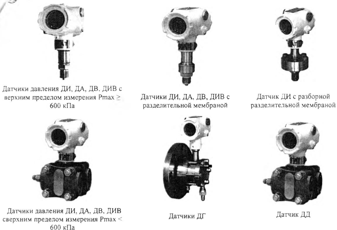
Рисунок 1 - Общий вид датчиков
