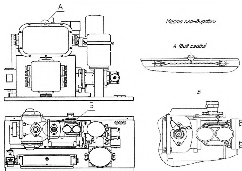
Рисунок 1 - Общий вид колонок топливораздаточных 1КЭД «Ливенка», 2КЭД «Ливенка»
