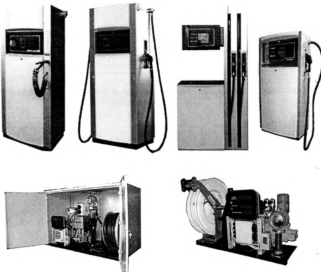
Рисунок 1 - Общий вид колонок топливораздаточных 1КЭД «Ливенка», 2КЭД «Ливенка»
