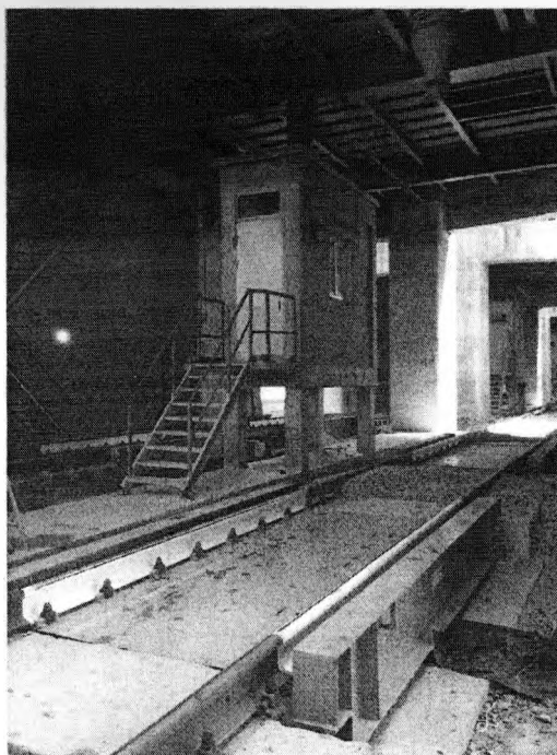
Рисунок 1 - Общий вид весов вагонных ВС-В
