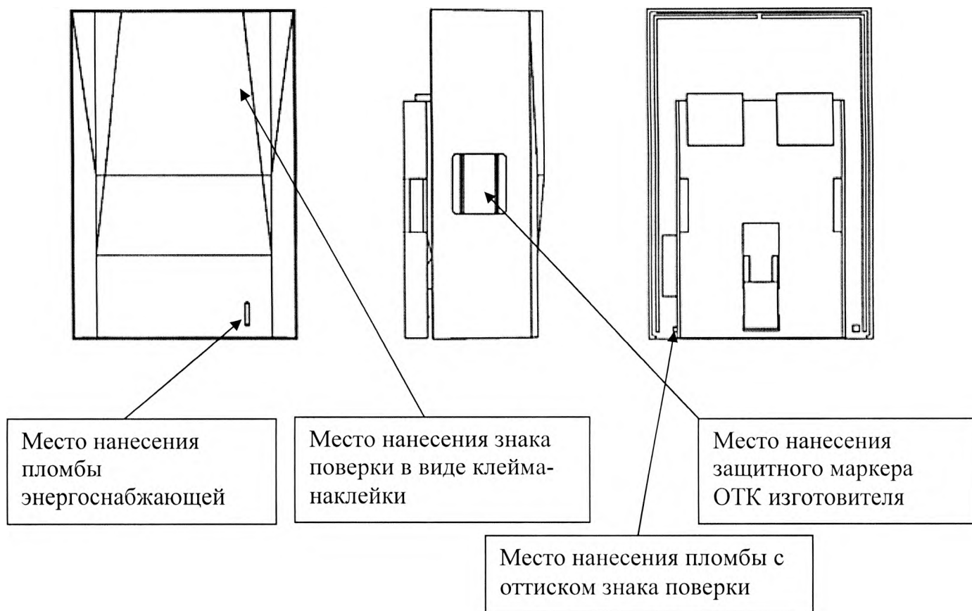
Рисунок А.2 – Места установки пломб и нанесения знака поверки для счетчиков в корпусе модификации SP2.
