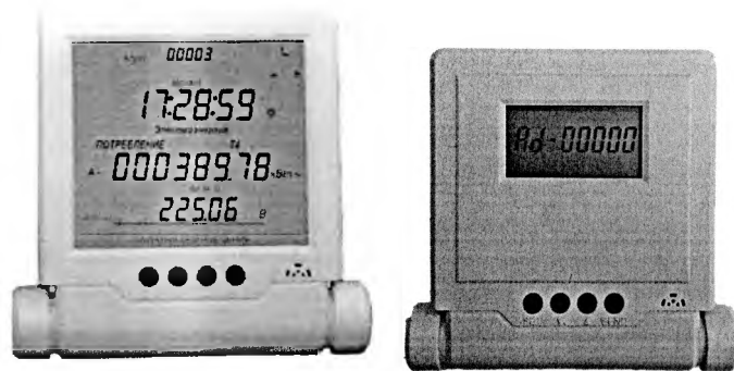
Рисунок 3 – Внешний вид выносных модулей отображения информации
