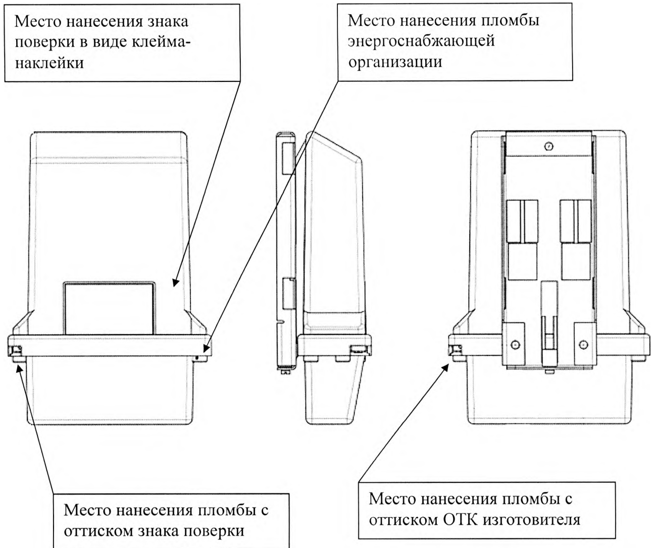
Рисунок А.1 – Места установки пломб и нанесения знака поверки для счетчиков в корпусе модификации SP1, SP3.
