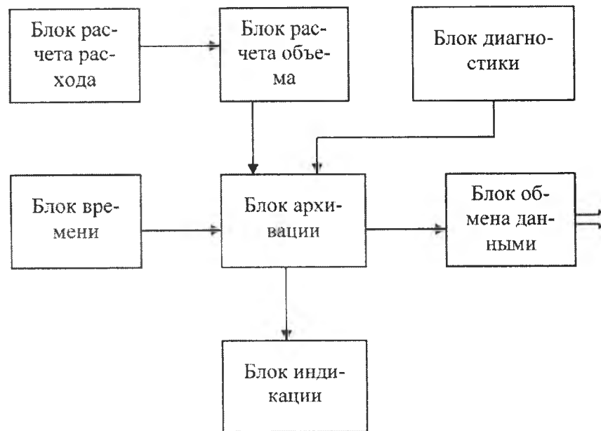
Рис. 3. Структура ПО
