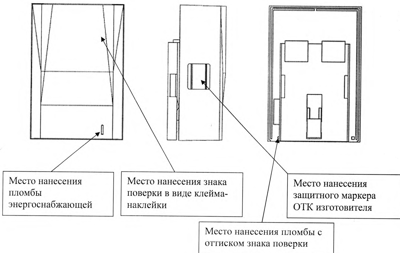
Рисунок Б.1 – Места установки пломб и нанесения знака поверки для счетчиков в корпусе модификации SP2.
