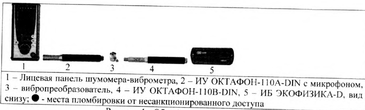
Рисунок 1 - Общий вид шумомера – виброметра
