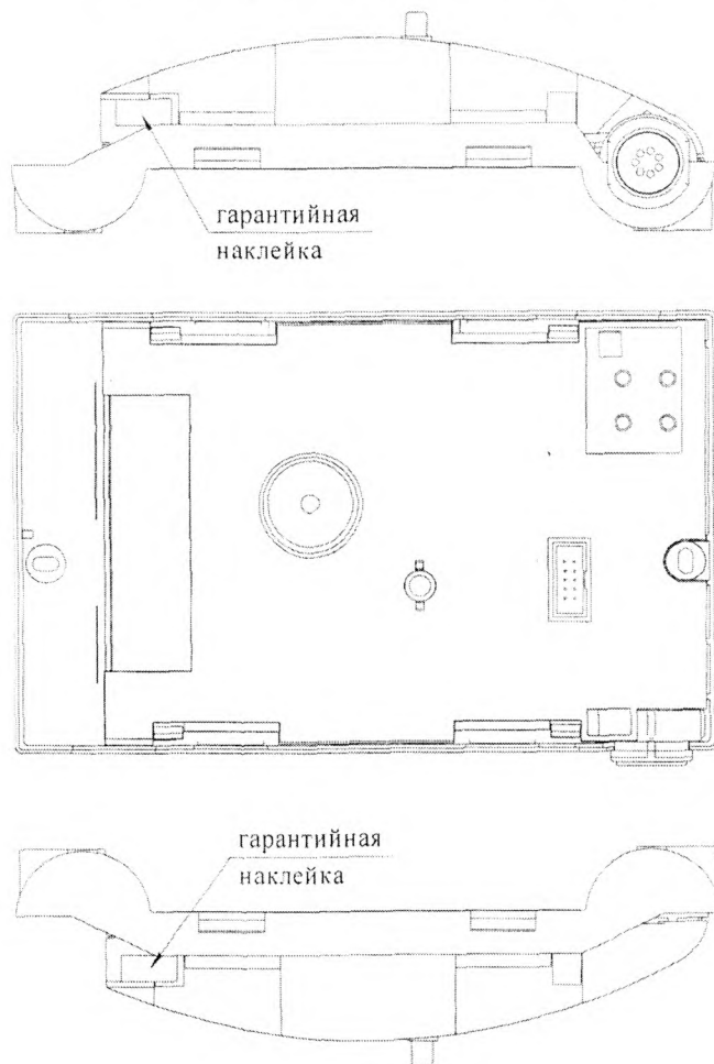
Рисунок 2 - Схема пломбировки сигнализаторов от несанкционированного доступа и обозначение мест для нанесения гарантийных наклеек
