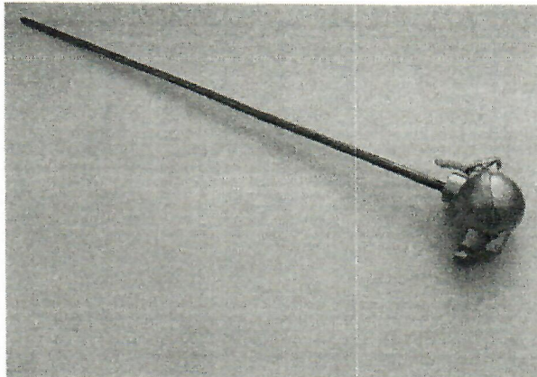
Рис.2 Модификация ТПП/ТПР-104
