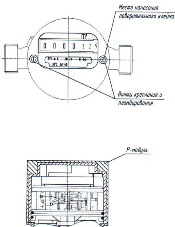
Рисунок 2А Схема пломбировки от несанкционированного доступа с указанием места для нанесения оттисков клейм для счетчиков ЕТК-м-ЗК и ЕТМ-м-ЗК
