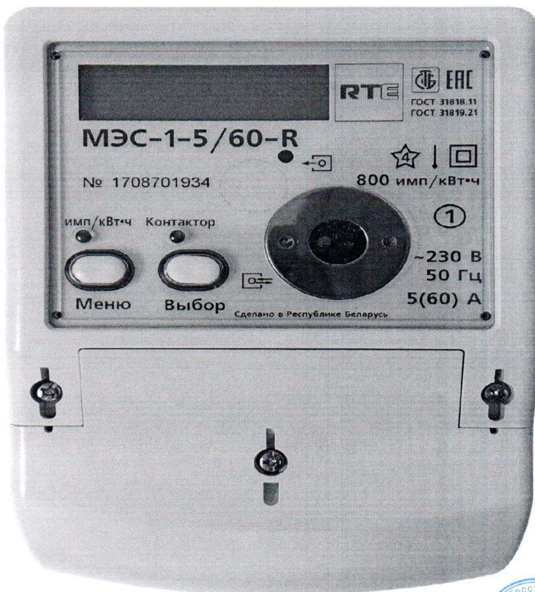
Рисунок 2 – Внешний вид счетчиков МЭС-1
