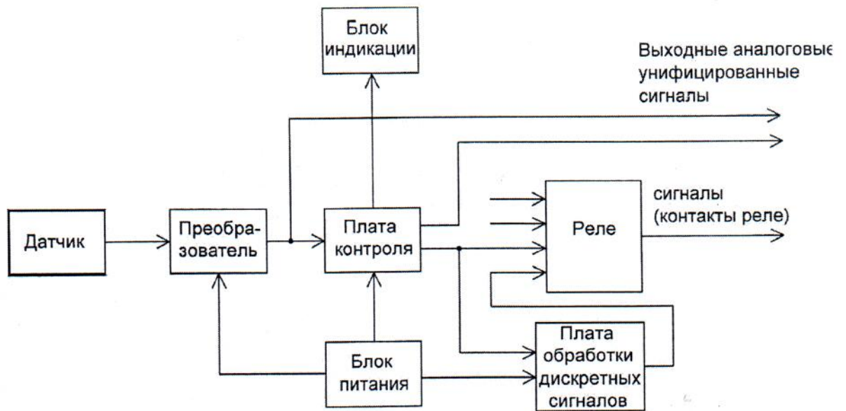
Рисунок 2 - Структурная схема
