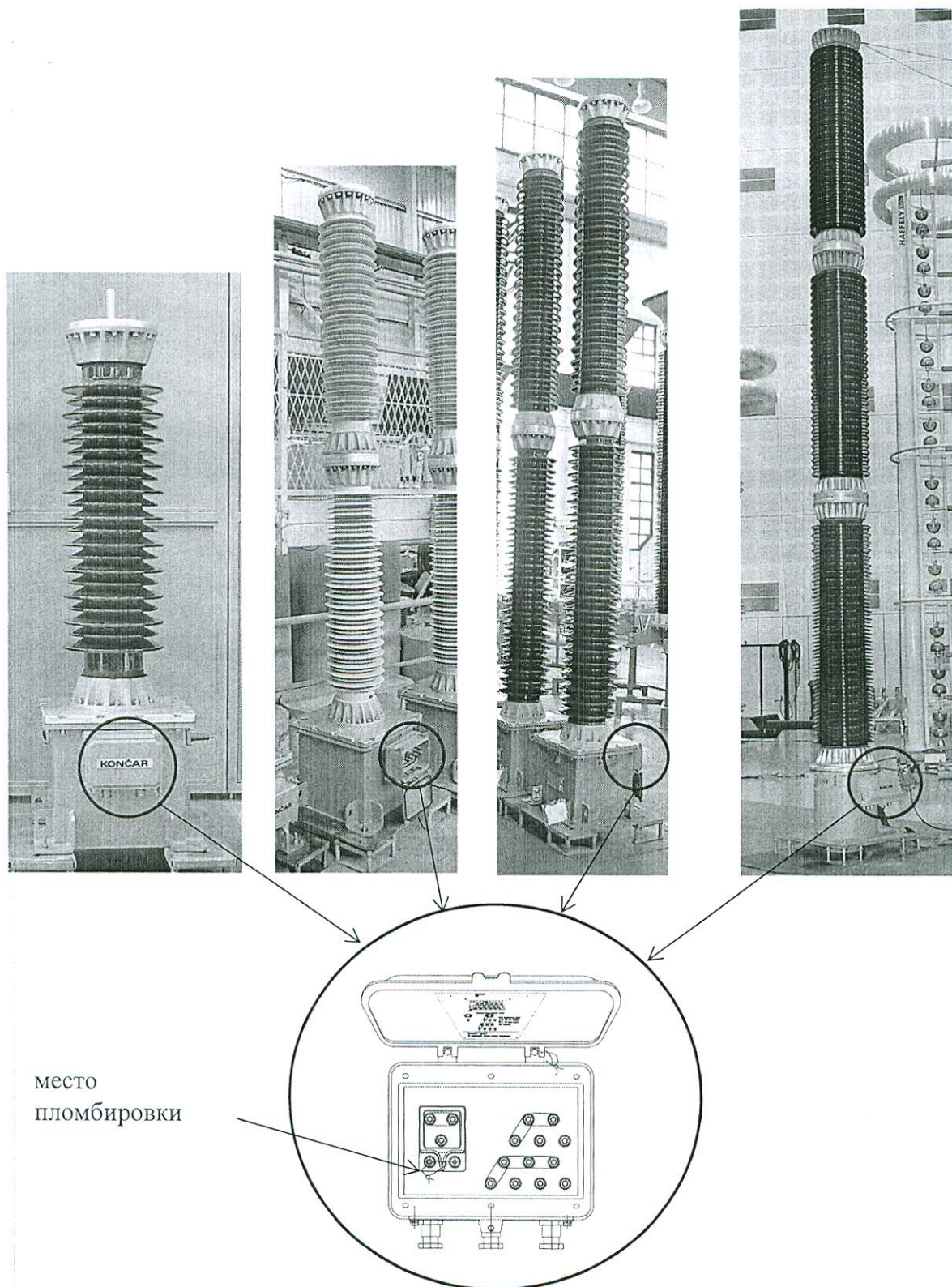
Рисунок 2 Схема пломбировки трансформаторов VCU-123, VCU-245, VCU-362, VCU-765
