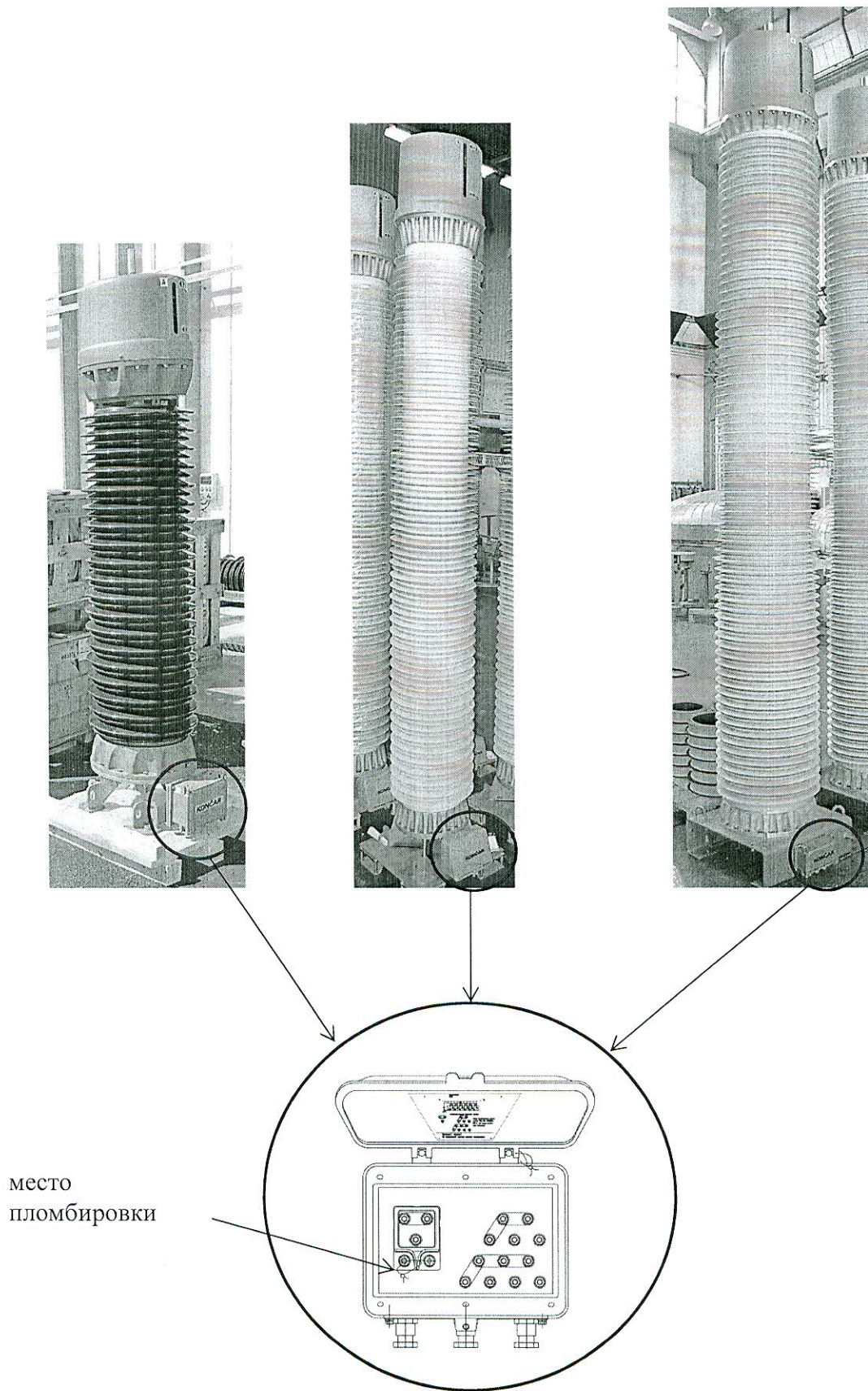
Рисунок 2 Схема пломбировки трансформаторов VPU-123, VPU-245, VPU-362
