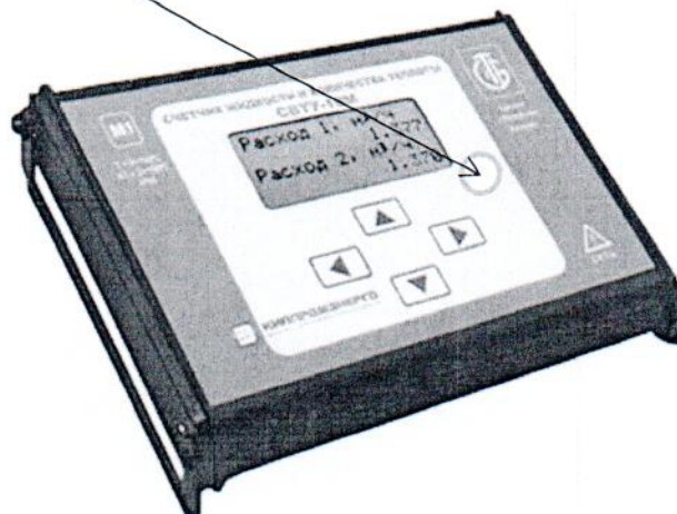
Рисунок А.1 - Место нанесения знака поверки в виде клейма – наклейки на счетчики жидкости и количества теплоты СВТУ-10М
