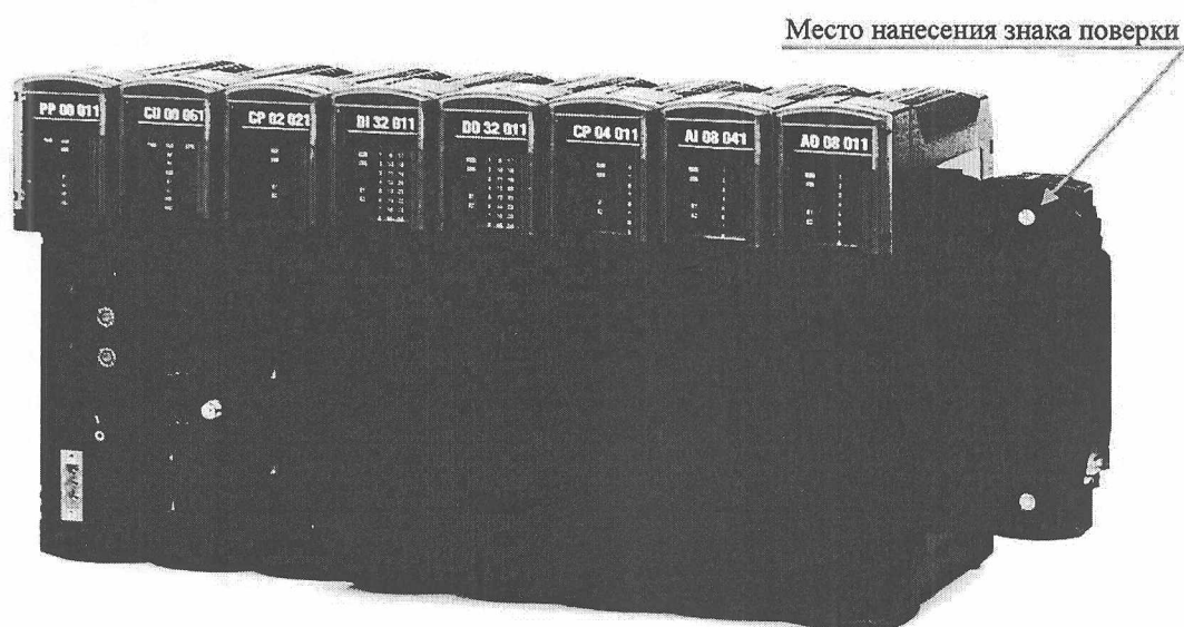
Рисунок 2 Общий вид и место нанесения знака поверки контроллера REGUL R500
