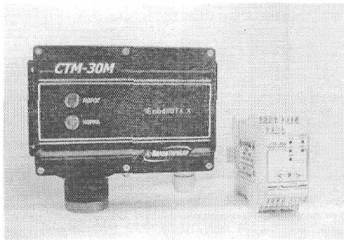
Рисунок 1а - Сигнализаторы СТМ-30М с диффузионным отбором пробы без цифровой индикации
