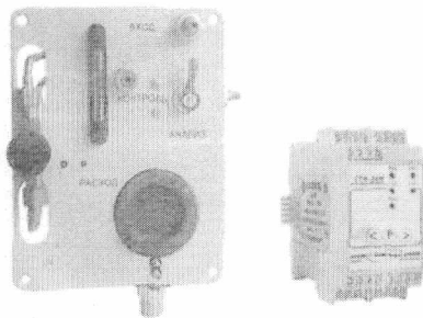
Рисунок 1д - Сигнализаторы СТМ-30М-10 с принудительным отбором пробы без цифровой индикации
