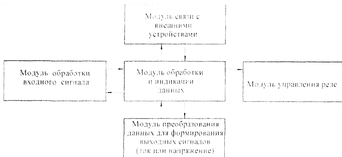
Рисунок 3 – Структура ПО.
