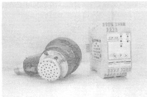
Рисунок 1в - Сигнализаторы СТМ-30М-10 с диффузионным отбором пробы без цифровой индикации
