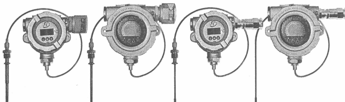
Рисунок 5 - Погружаемые кабельные взрывозащищенные ППТСК/Exd/ИНД, ППТСК/Exdi/ИНД
