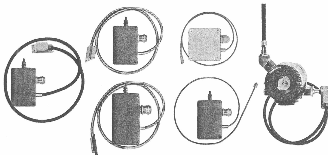
Рисунок 8 - Поверхностные общепромышленные ППТП/Оп и взрывозащищенные ППТП/Ех с корпусами типов «К3М» - «К7»
