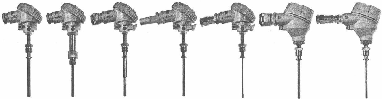
Рисунок 1 - Погружаемые общепромышленные ППТС/Оп и взрывозащищенные ППТС/Exi, ППТС/Exd, ППТС/Exdi
