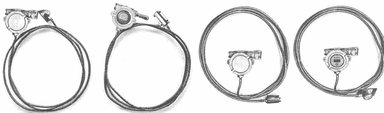
Рисунок 10 - Поверхностные общепромышленные ППТП/Op, ППТП/Op/ИНД и взрывозащищенные ППТП/Exd, ППТП/Exdi, ППТП/Exd/ИНД, ППТП/Exdi/ИНД с корпусами типов «К1», «К2»
