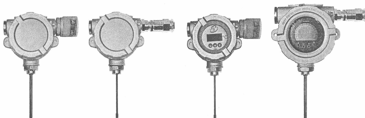
Рисунок 7 - Взрывозащищенные ППТСП/Ехd, ППТСП/Ехdi, ППТСП/Ехd/ИНД, ППТСП/Ехdi/ИНД для измерения температуры окружающей среды (воздуха)
