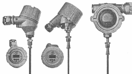
Рисунок 2 - Погружаемые общепромышленные ППТС/Оп/ИНД и взрывозащищенные ППТС/Exd/ИНД, ППТС/Exi/ИНД, ППТС/Exdi/ИНД
