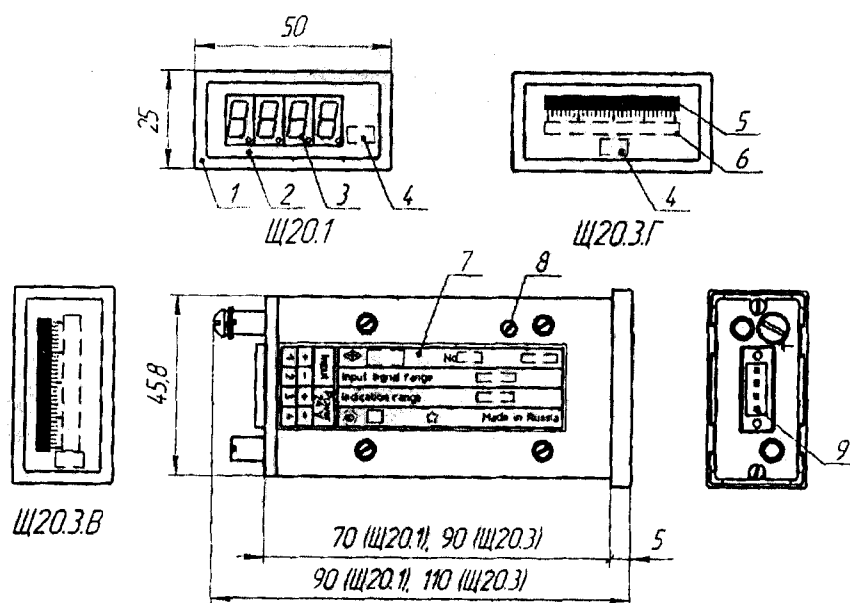
Рисунок 2 – Общий вид приборов Щ20
