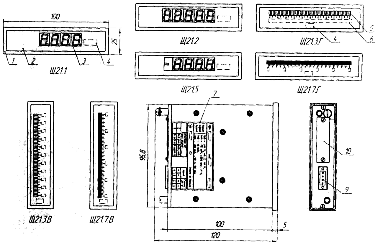
Рисунок 3 – Общий вид приборов Щ21
