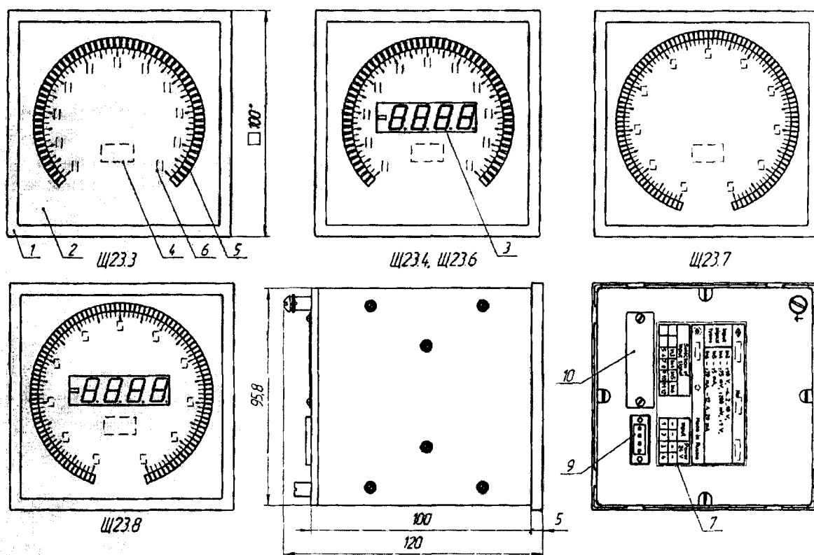
Рисунок 5 – Общий вид приборов Щ23
