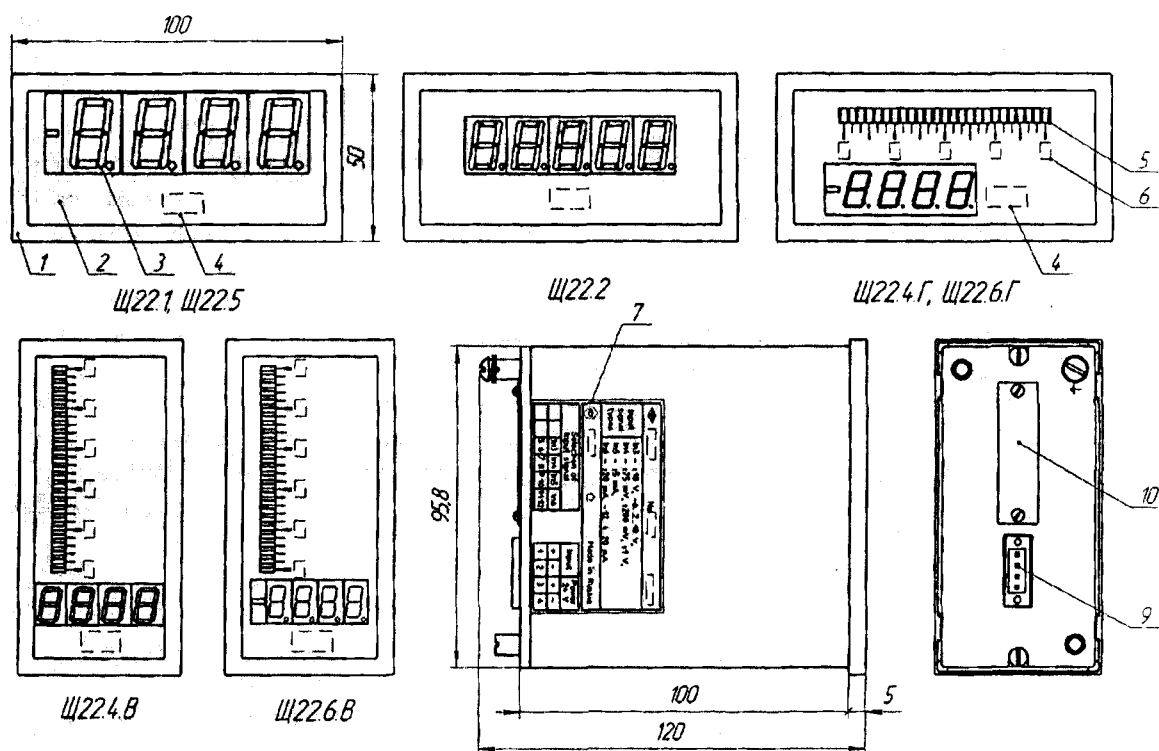
Рисунок 4 – Общий вид приборов Щ22
