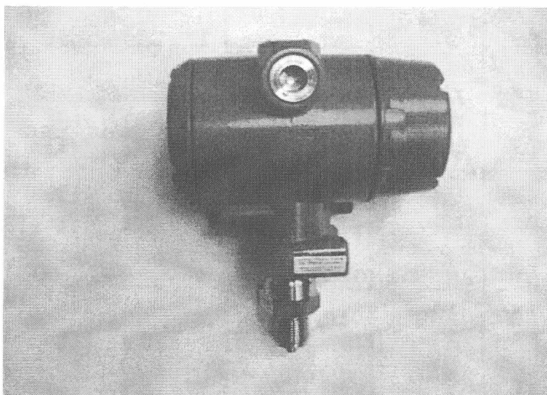
Рисунок 1 – Общий вид датчиков давления Метран-75
