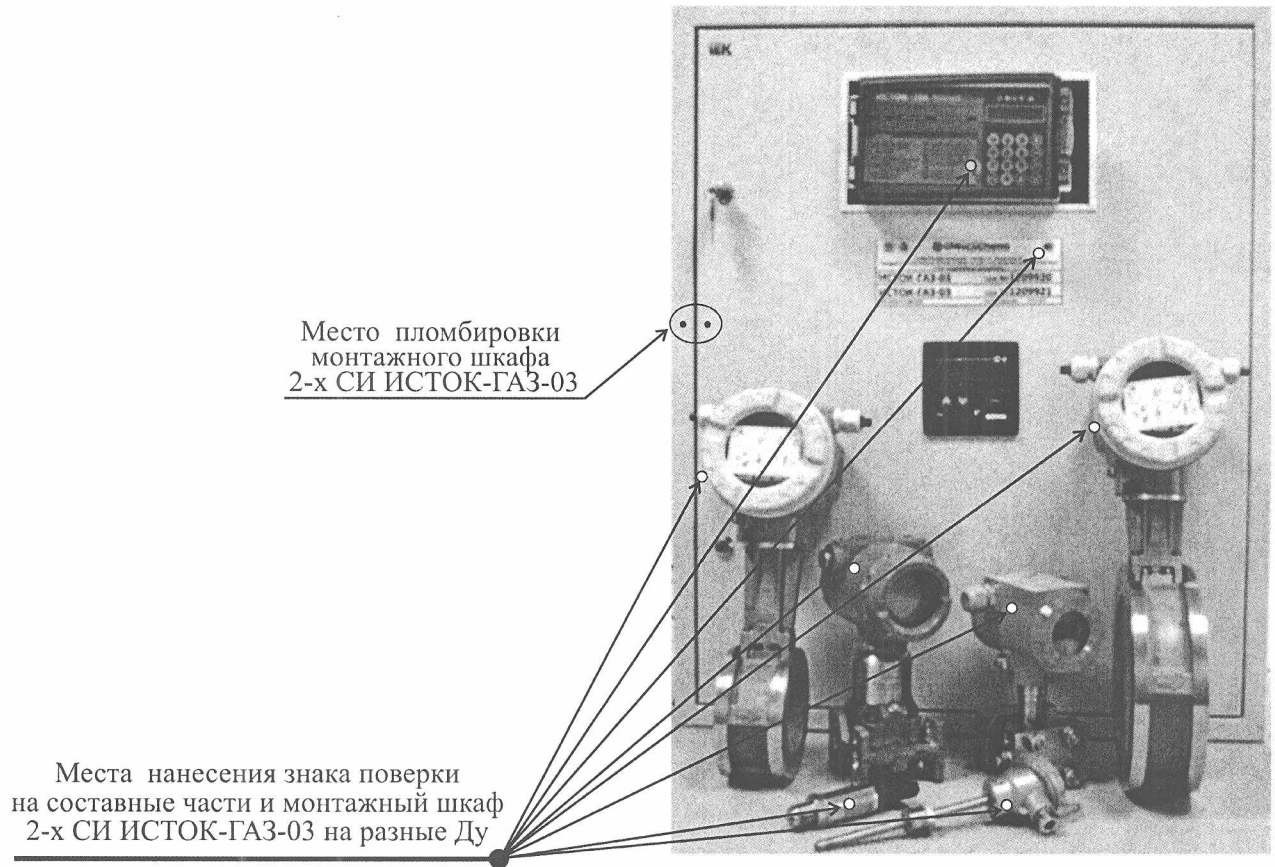
Рисунок А.1 - Места нанесения знака поверки на составные части и монтажный шкаф СИ ИСТОК и место пломбировки монтажного шкафа СИ ИСТОК на примере конкретного комплекта поставки (две СИ ИСТОК-ГАЗ-03 с расходомерами на разные Ду)
