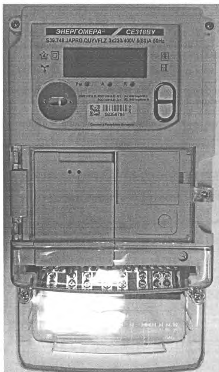
Рисунок 2 – Внешний вид счетчиков электрической энергии CE318BY, корпус S39
