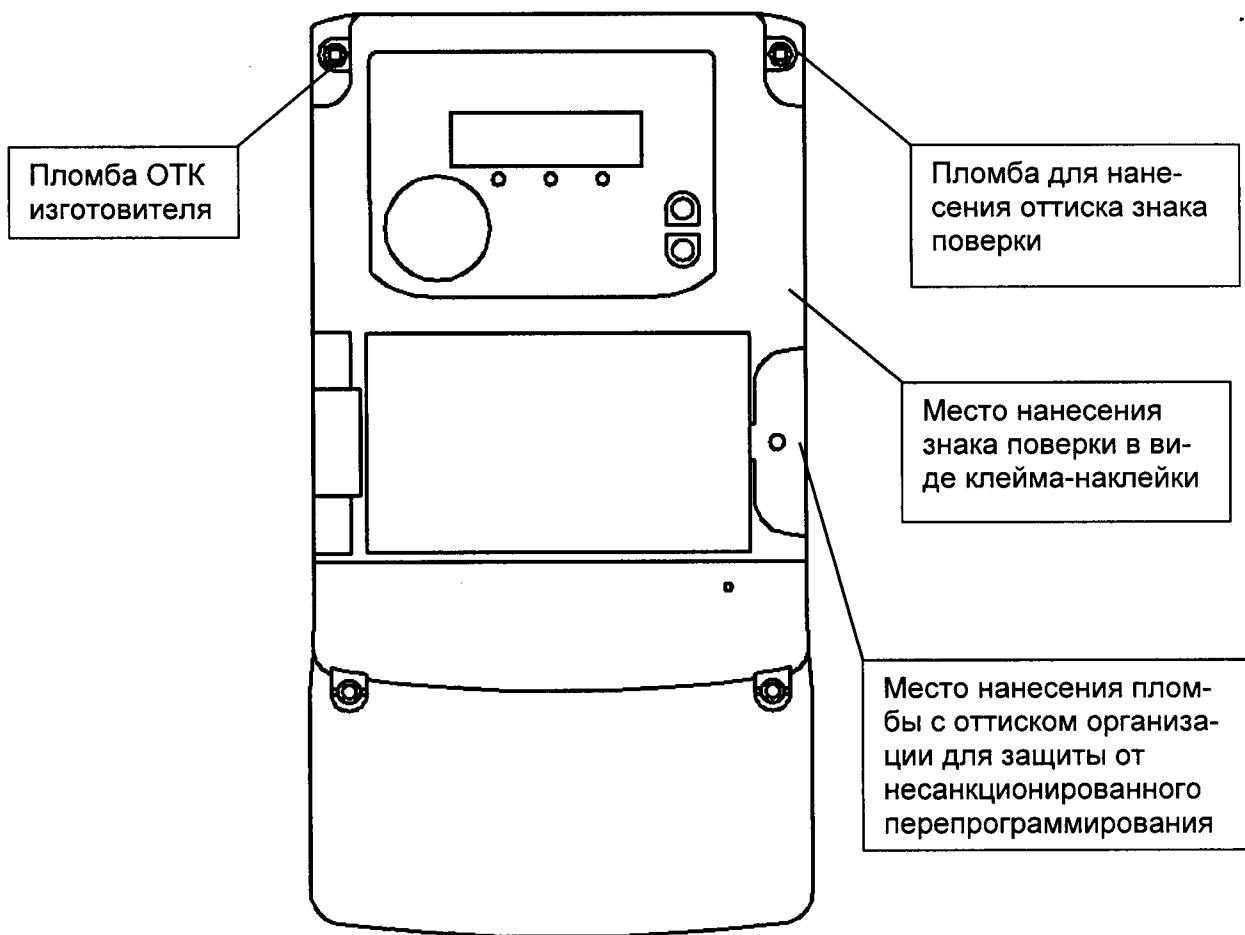
Рисунок А.3 – Корпус счетчиков CE318BY S39
