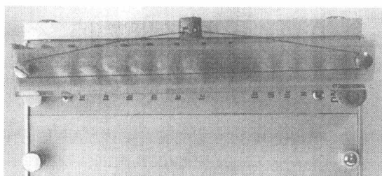
Рисунок 9. Пломбировка клеммных соединителей измерительных цепей
