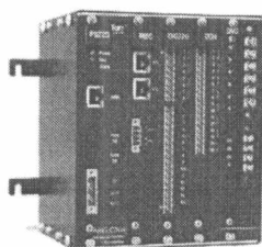
Рисунок 5. Общий вид контроллера ARIS C304, вид спереди
