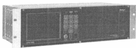
Рисунок 1. Общий вид контроллера ARIS C303, вид спереди
