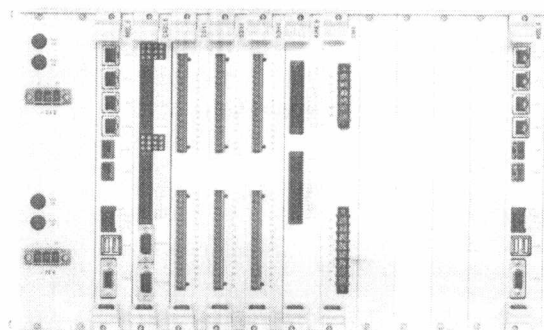
Рисунок 8. Общий вид контроллера ARIS C306, вид сзади
