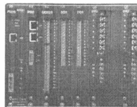
Рисунок 6. Общий вид контроллера ARIS C305, вид спереди
