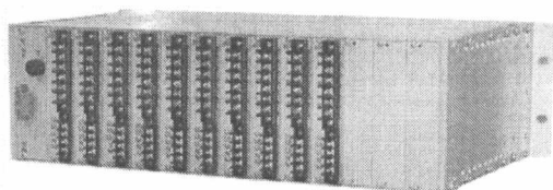
Рисунок 7. Многофидерный измеритель (счетчик электроэнергии), вид сзади
