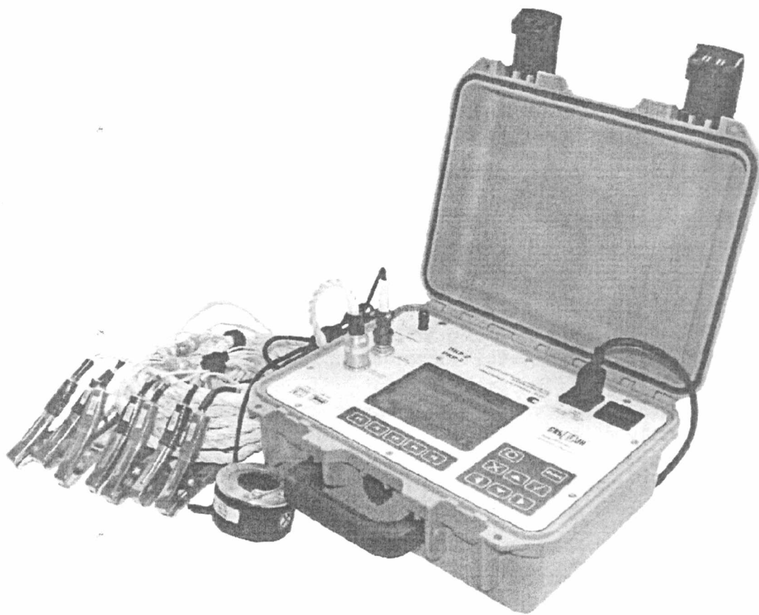
Рис. 2 Измерительный блок
