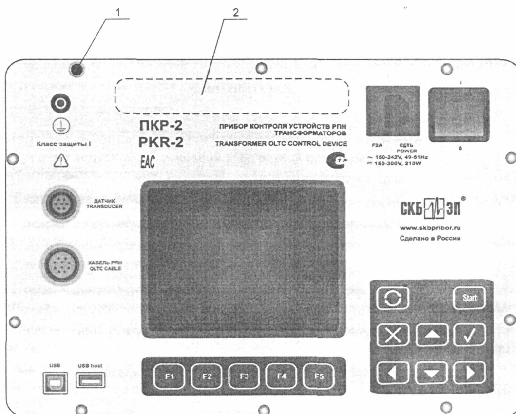
Рис. 3 Схема панели
