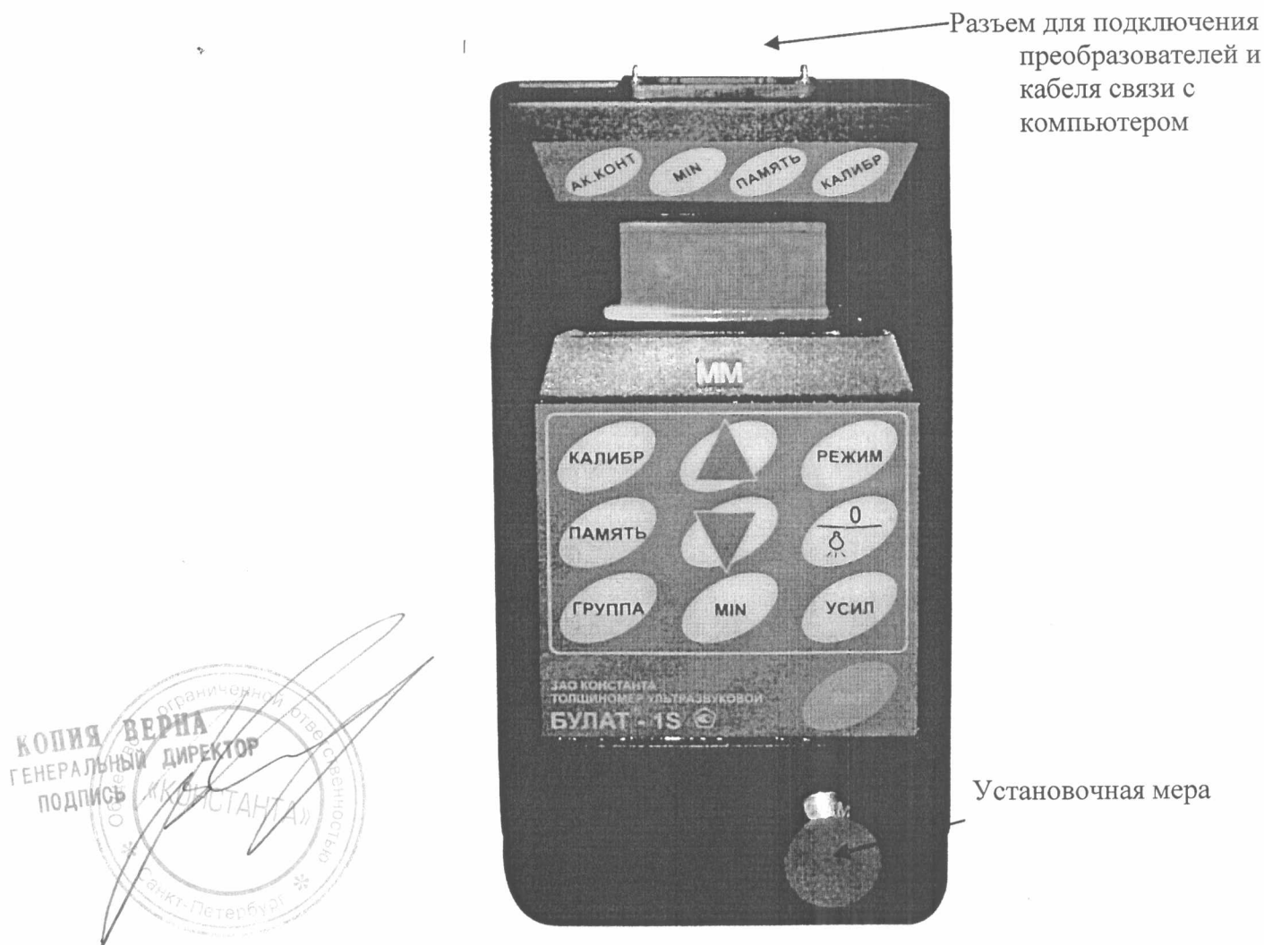
Рисунок 1. Блок обработки информации
