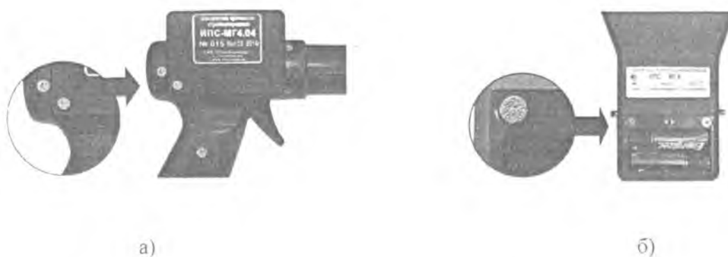
Рисунок 2 – Обозначение места для нанесения отиска клейма
